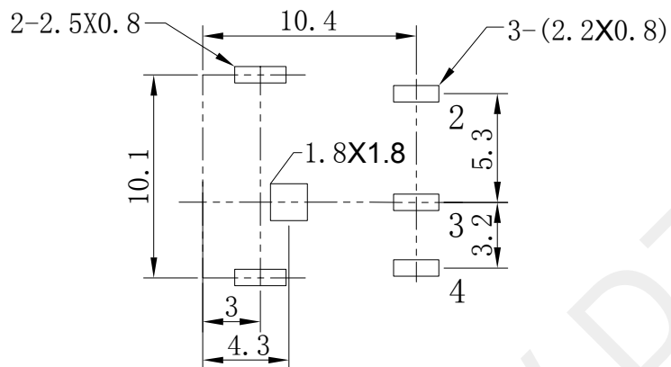
线路板开孔尺寸 P.C.B LAYOUT
